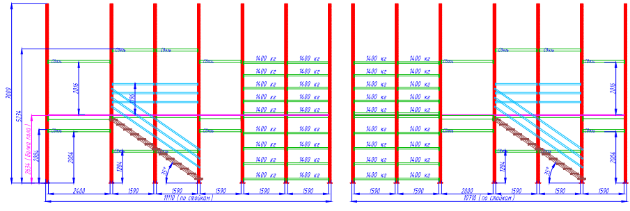
В-В
